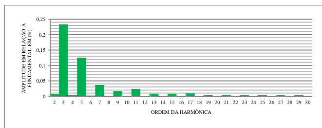
Fig. 4. Espectro de harmônicas na corrente da fase S
