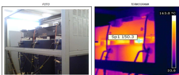
Fig. 1. Análise termográfica do transformador
